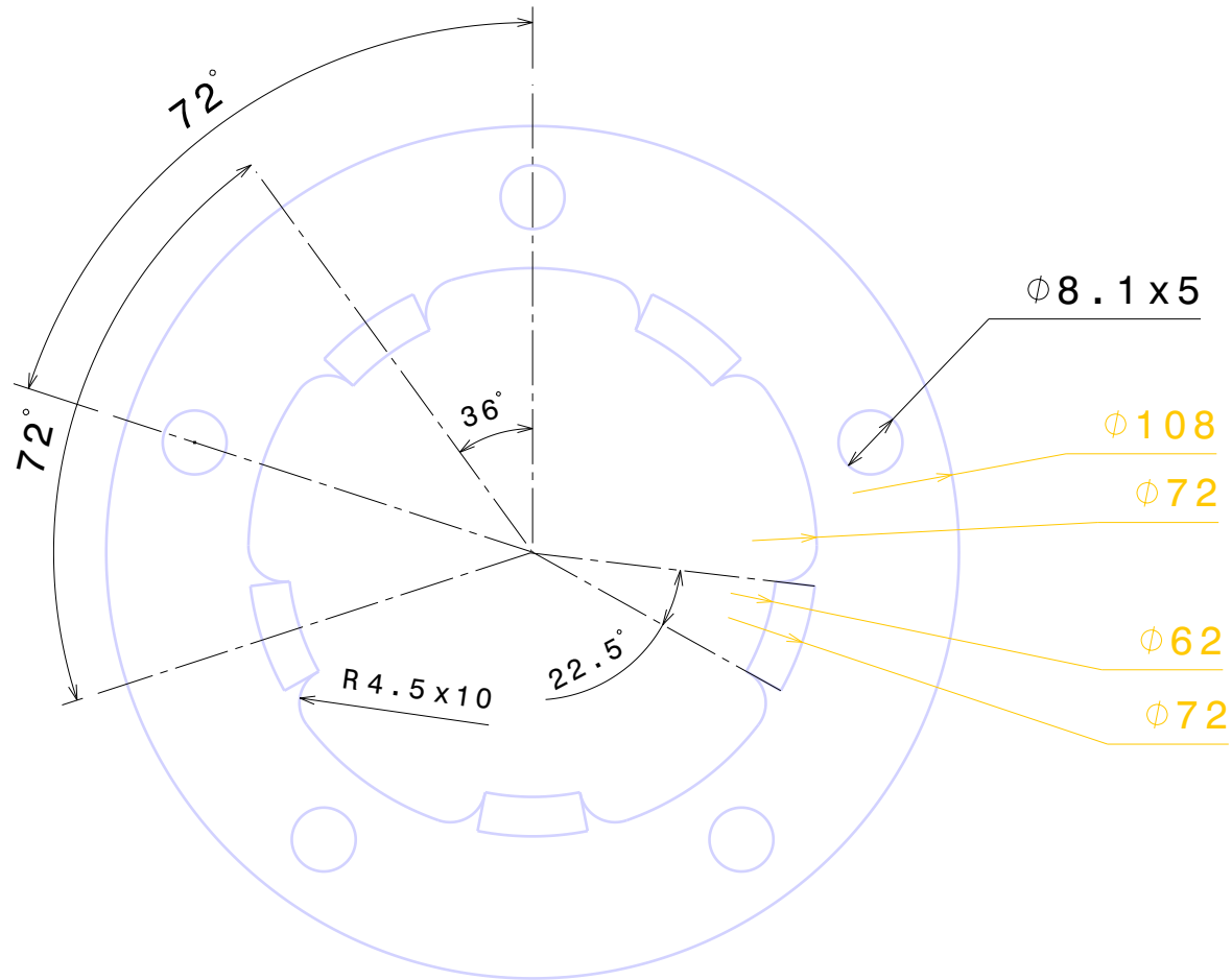
Front view Scale: 1:1
