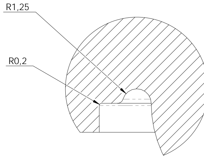
DÉTAIL B ECHELLE 5 : 1
