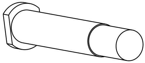
Vue isométrique Echelle : 1:1
