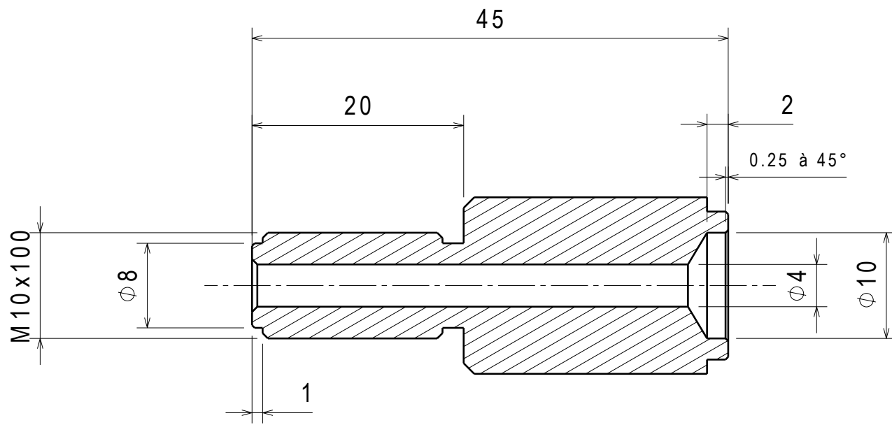
Coupe A-A
