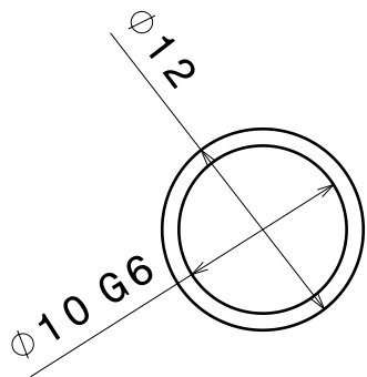
Vue de face Echelle : 2:1
