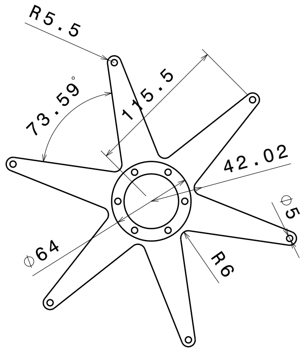
Vue de face Echelle : 1:3
