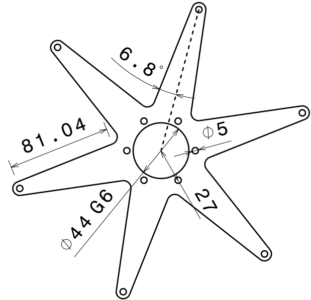
Vue de derrière Echelle : 1:3
