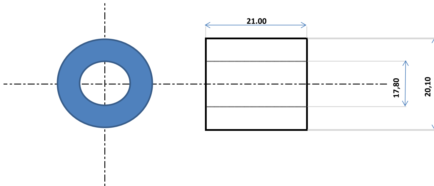
Bague en Bronze ou similaire pour axe de béquille latérale DUCATI 900 MOSTRO Cotes en mm
