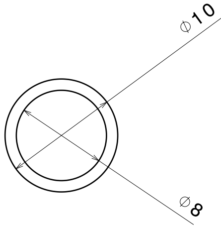
Vue de face Echelle : 3:1
