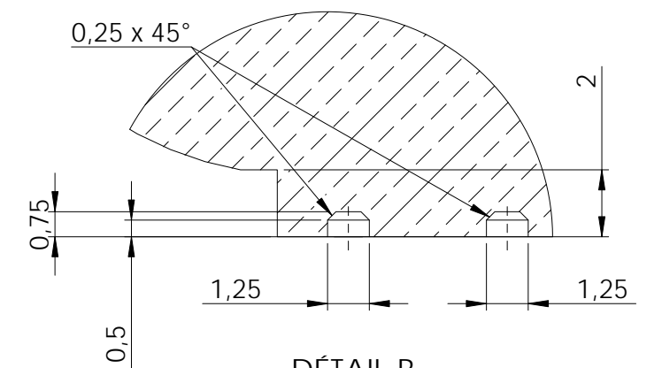
DÉTAIL B ECHELLE 5 : 1
