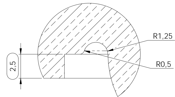
DÉTAIL A ECHELLE 5 : 1
