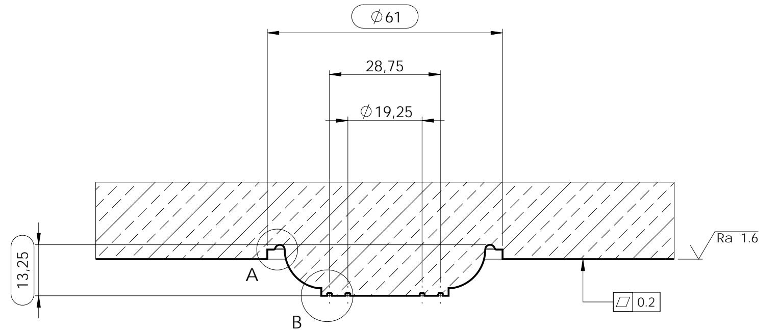
COUPE A-A
