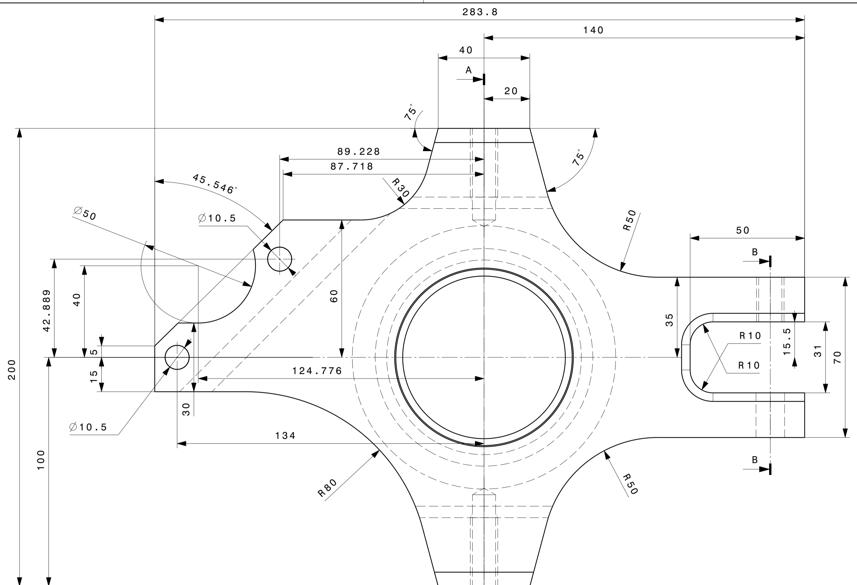
Vue de face Echelle : 1:1
