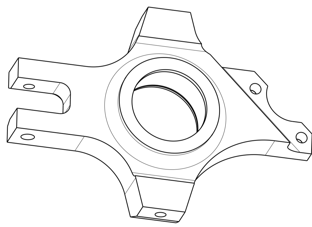
Vue isométrique Echelle : 1:2
