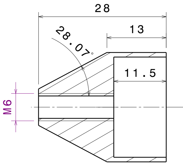
Coupe A-A Echelle : 2:1
