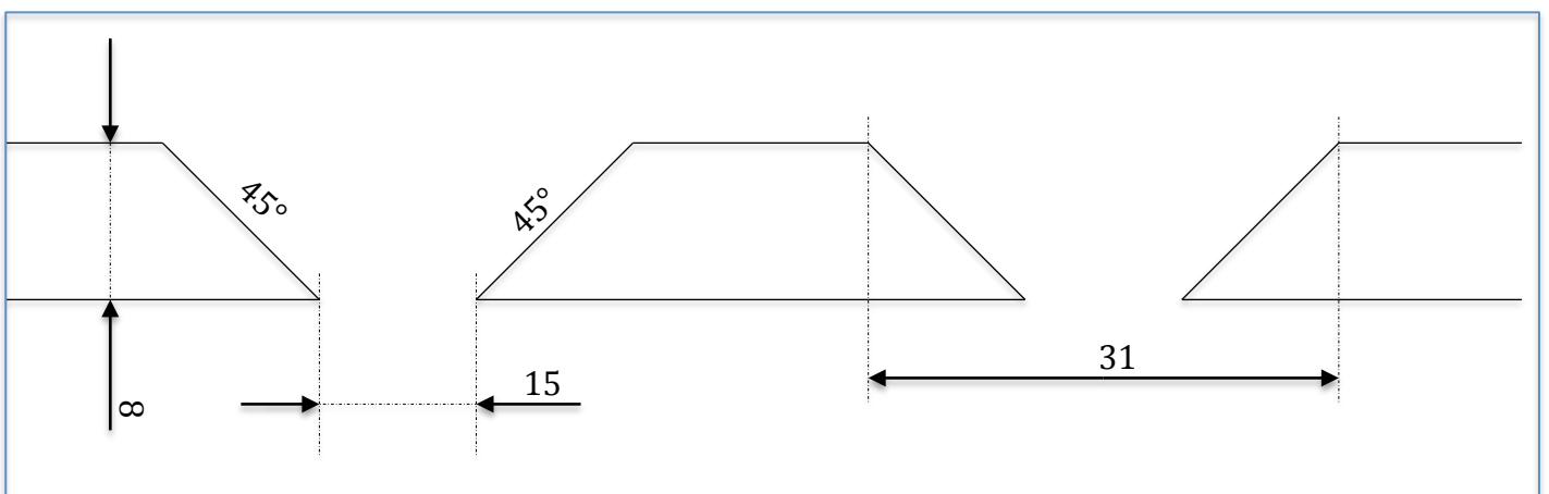
Vue coupe
