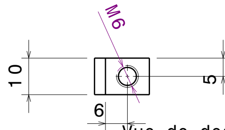
Vue de dessus Echelle : 1:1
