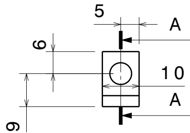
Vue de gauche Echelle : 1:1
