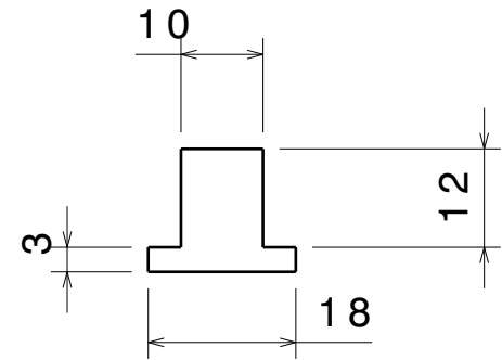
Vue de derrière Echelle : 1:1
