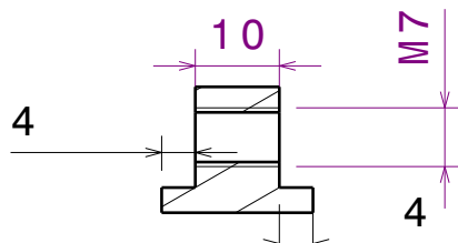
Coupe A-A Echelle : 1:1
