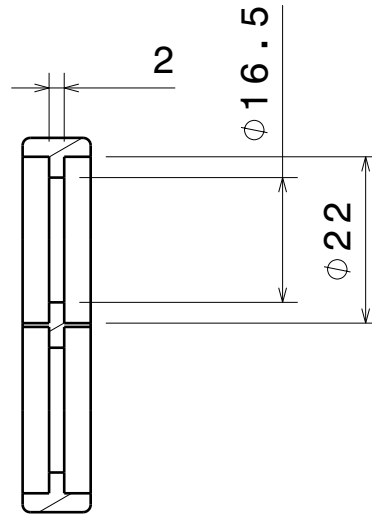
Coupe A-A Echelle : 1:1
