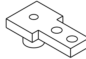
Vue isométrique Echelle : 1:1
