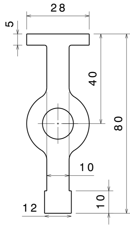
Vue de face Echelle : 1:1
