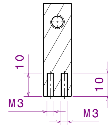
Coupe B-B Echelle : 1:1
