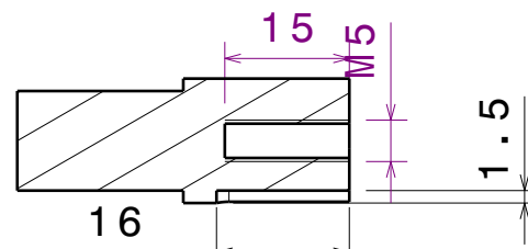
Coupe A-A Echelle : 1:1
