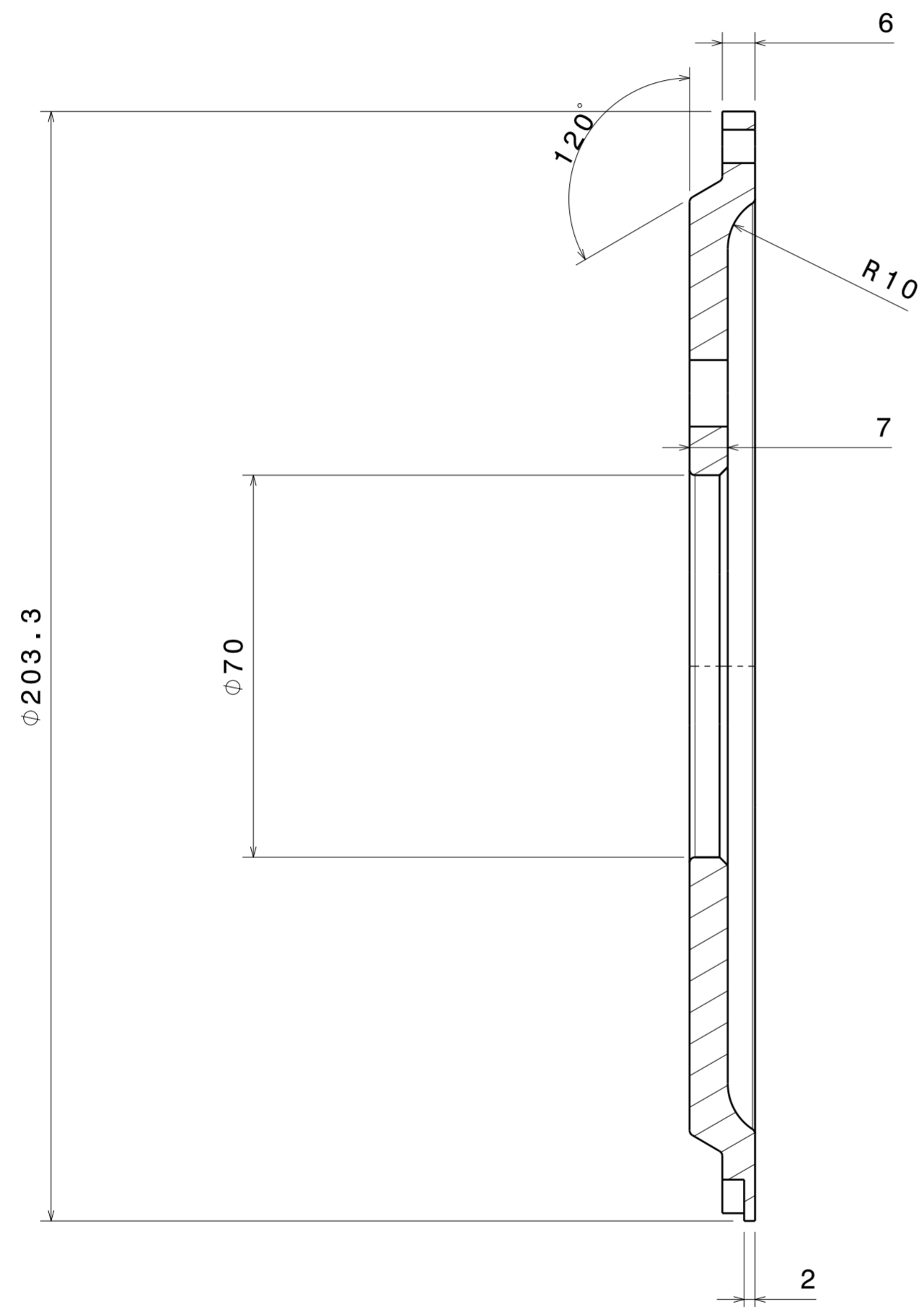
Coupe A-A Echelle : 1:1
