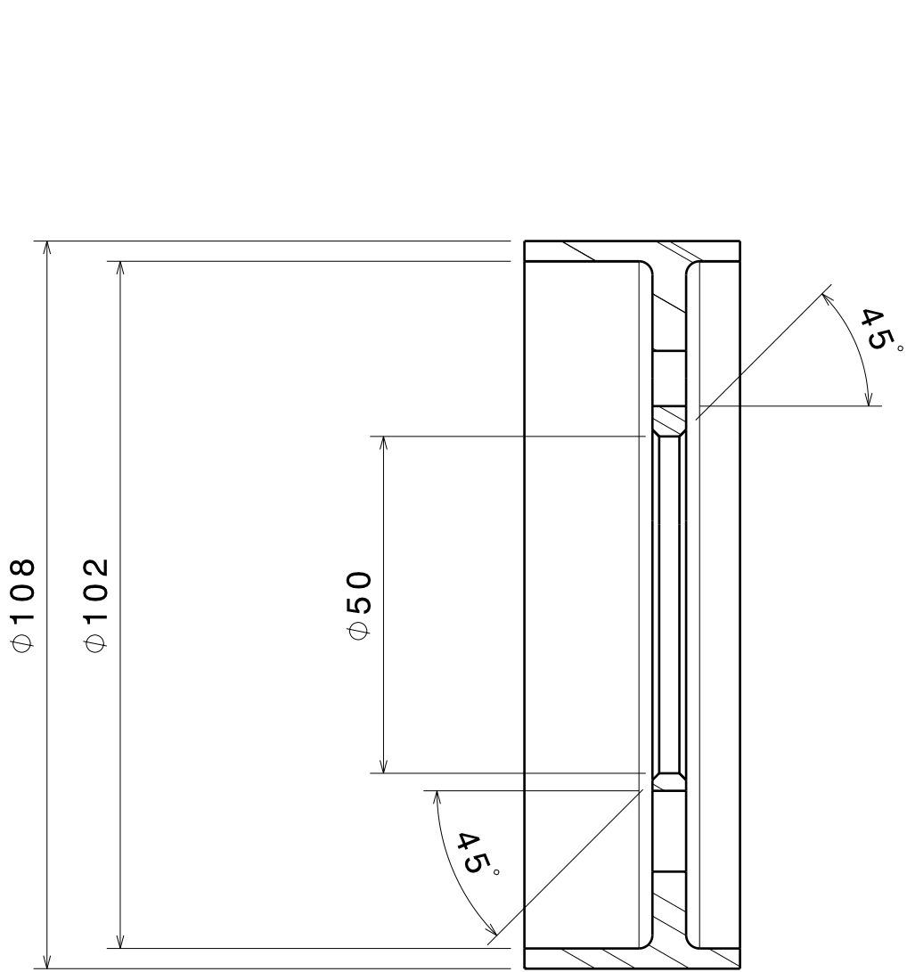
Coupe A-A Echelle : 1:1
