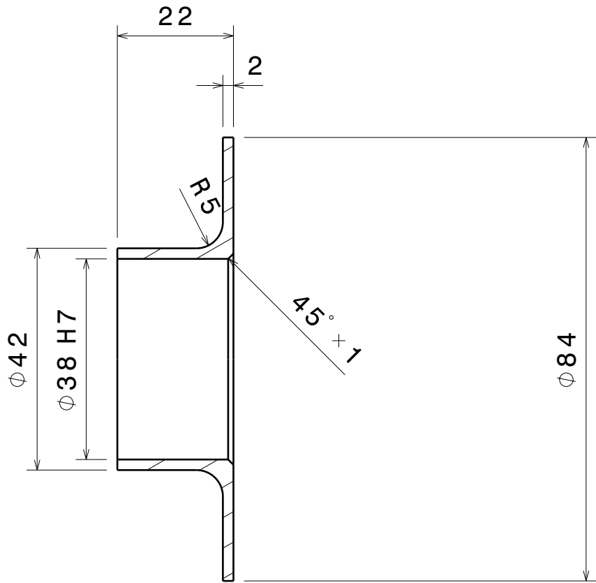
Coupe A-A Echelle : 1:1
