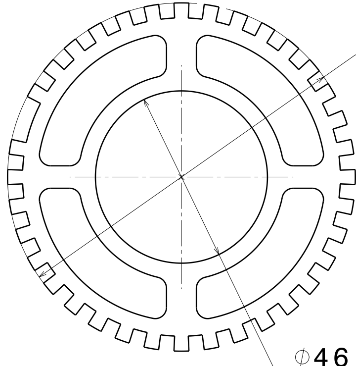
Vue de face Echelle : 1:1
