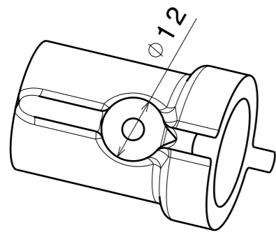
Vue auxiliaire C Echelle : 1:1
