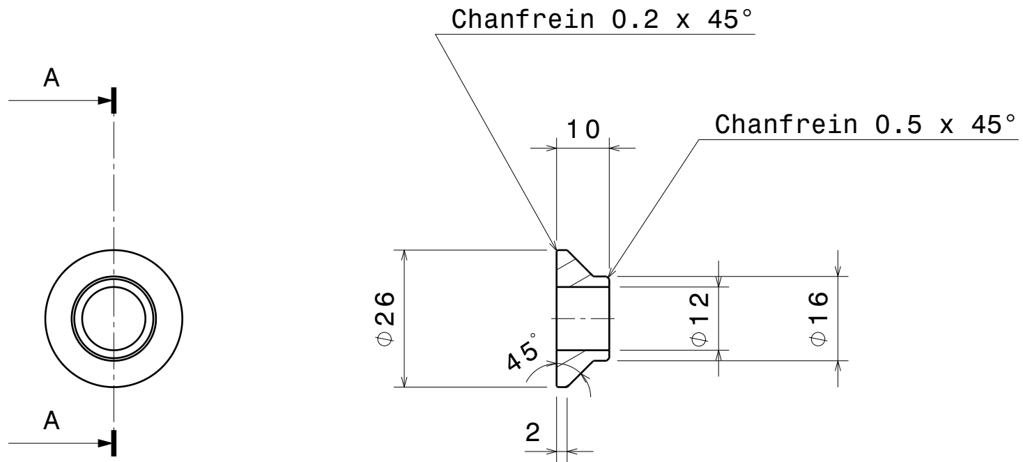
Vue de face Echelle : 1:1
