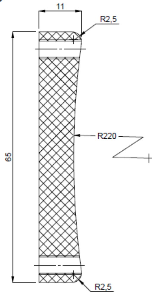
COUPE A-A
