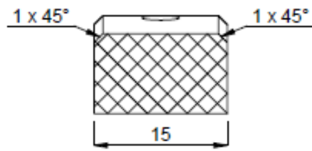
COUPE B-B
