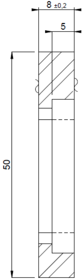
COUPE A-A
