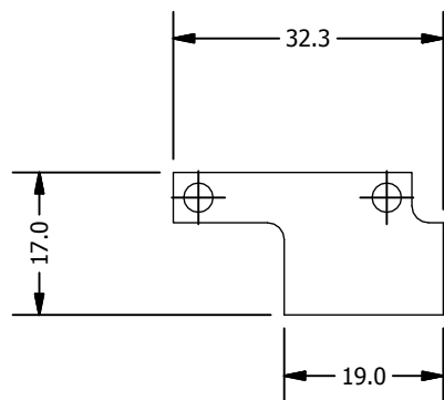
Front-View SCALE 1 : 1
