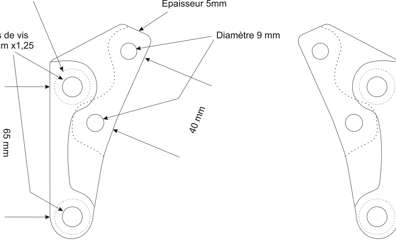
PLATINE DROITE
