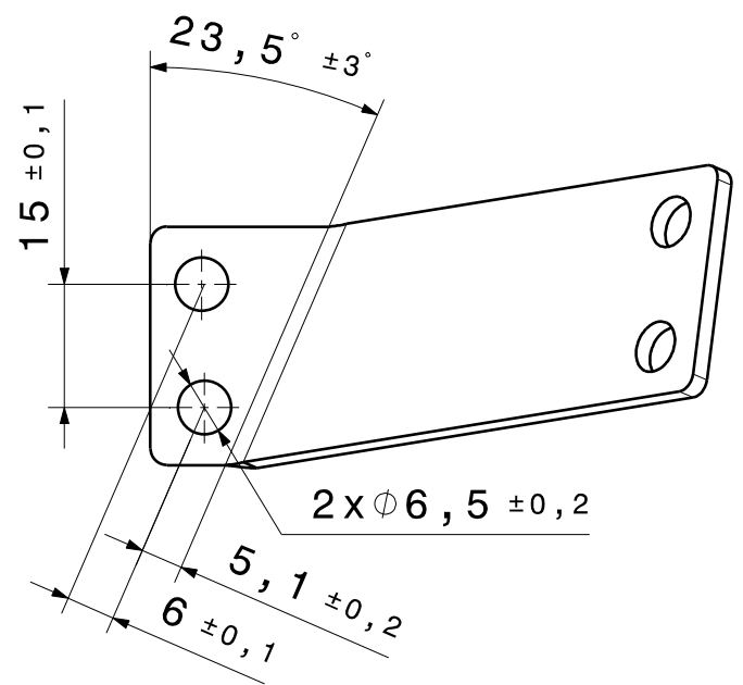
Vue de face Front view
