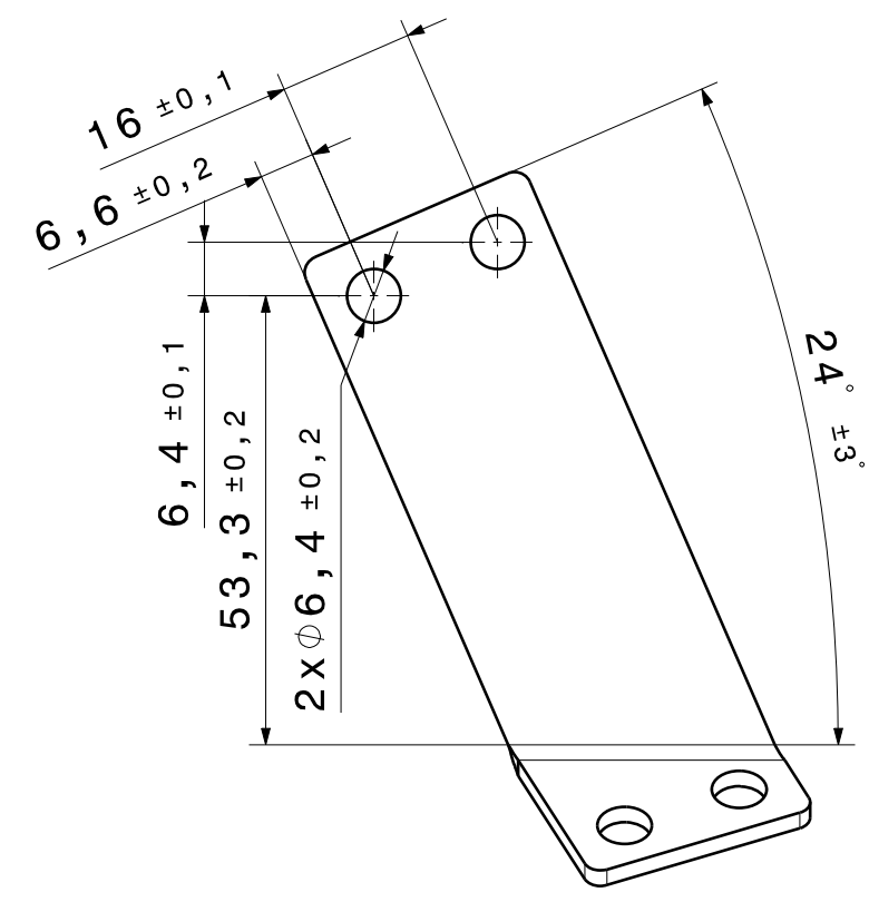
Vue de gauche Left view
