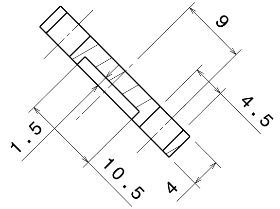
Coupe A-A
