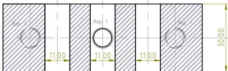
Coupe BB
