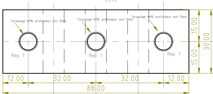
Coté
