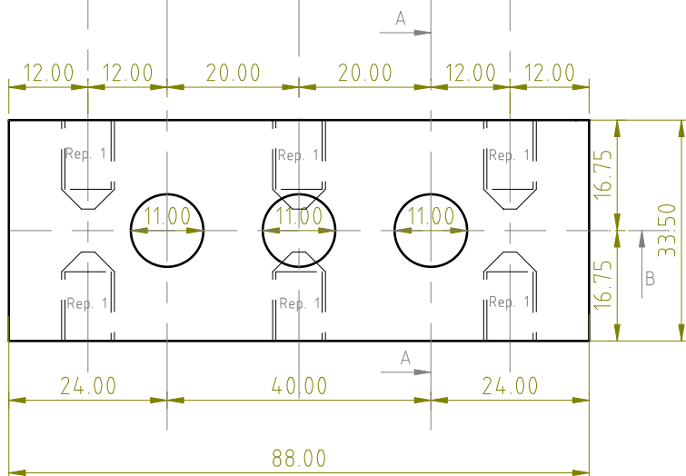
Dessus
