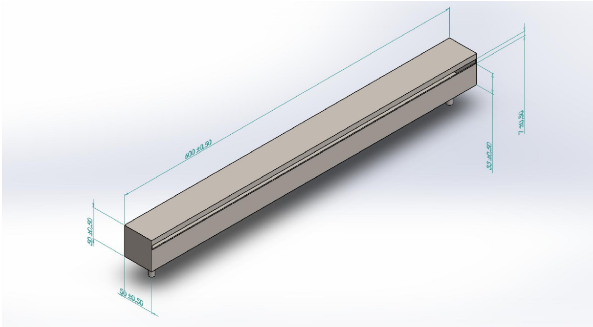
Figure 3 : vue en perspective (dimensions en mm, profondeur de la rainure de 25mm, comme sur la pièce 1)
