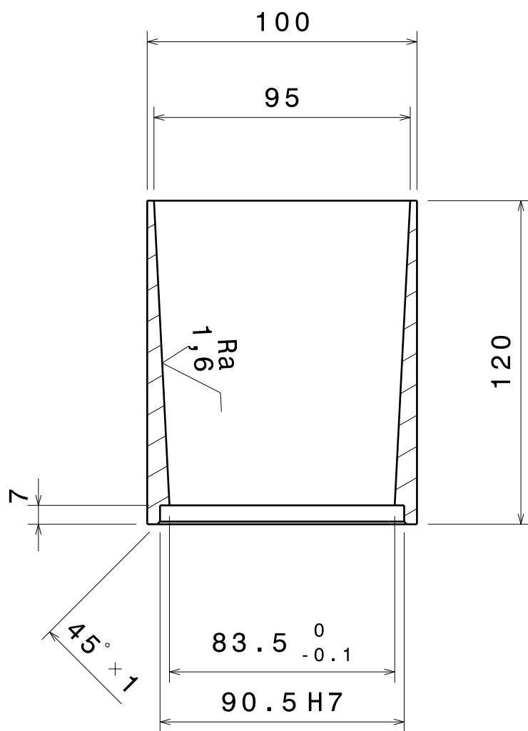
Coupe A-A Echelle : 1:2
