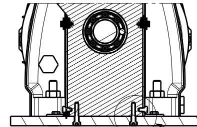
Coupe A-A Echelle : 1:4
