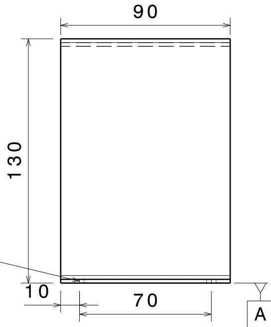
Vue de face Echelle : 1:2
