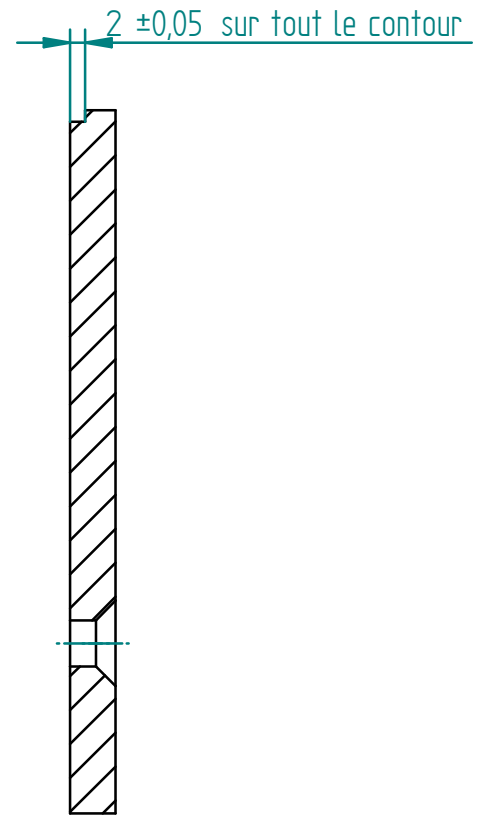
SECTION A-A
