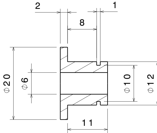
Coupe A-A Echelle : 2:1
