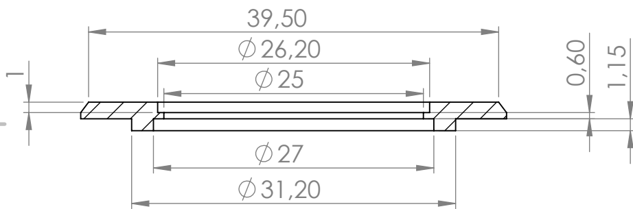
COUPE A-A ECHELLE 2 : 1
