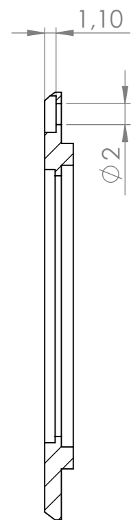
COUPE C-C ECHELLE 2 : 1
