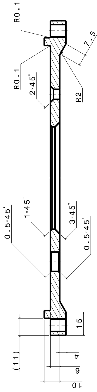
A-A Echelle : 2:1
