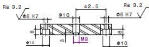
Coupe B-B Echelle : 1:1
