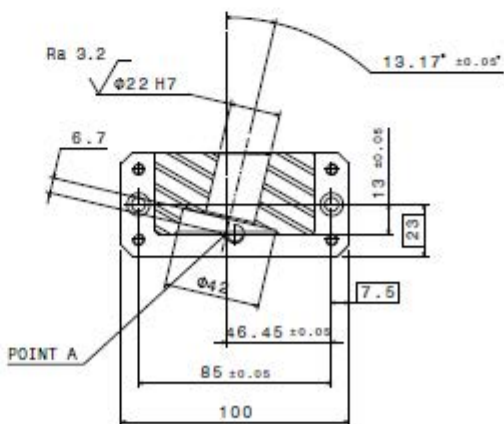
Coupe A-A Echelle : 1:1
