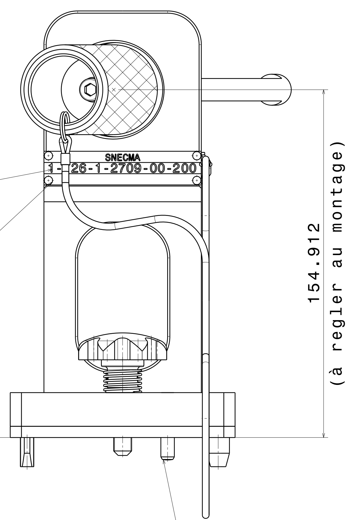
Dessus marbre Outillage de fraisage
