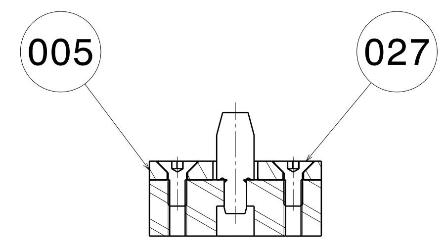
Coupe C-C Echelle : 1:1
