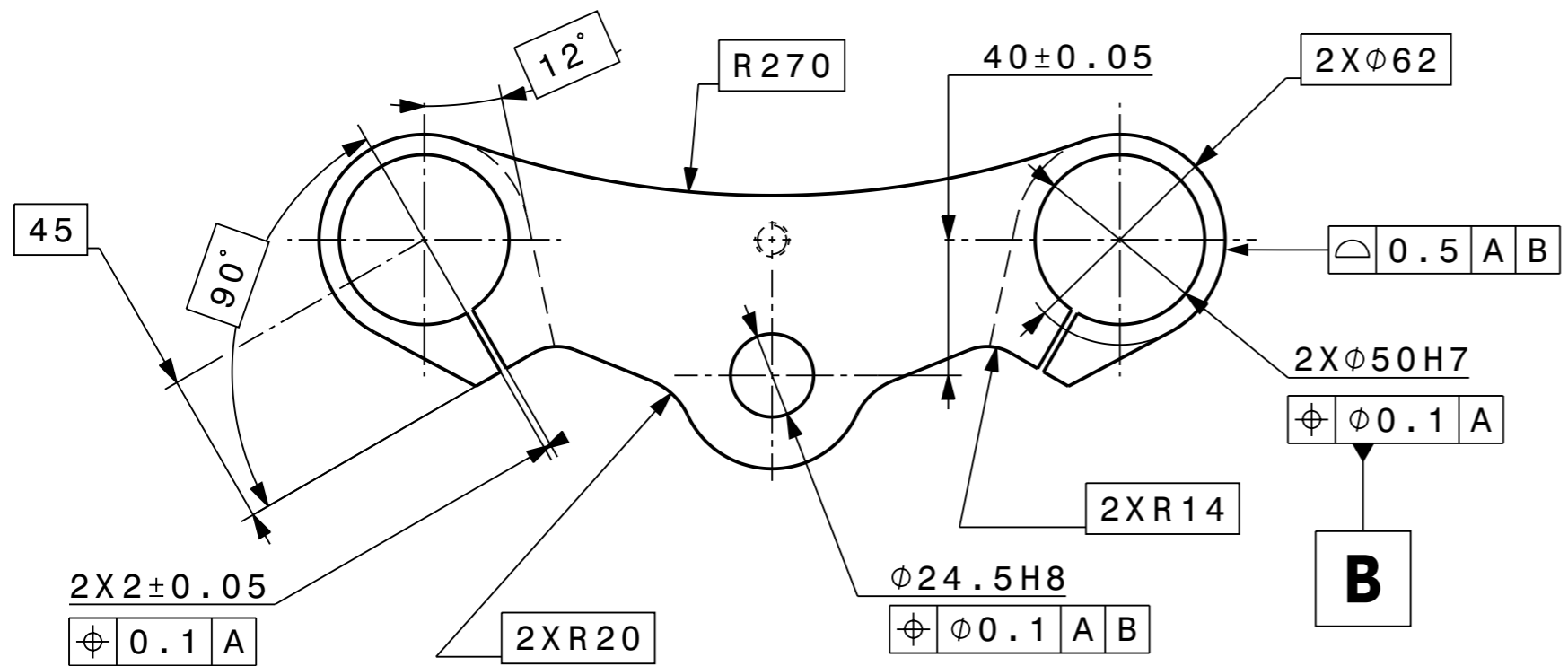
Vue de dessus 1:2
