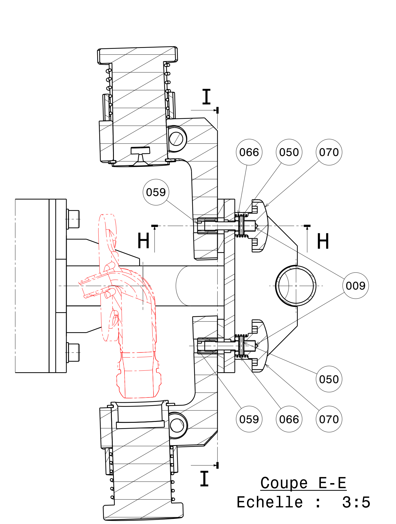
Coupe E-E Echelle : 3:5
