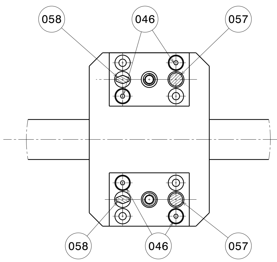
Coupe I-I Echelle : 3:5
