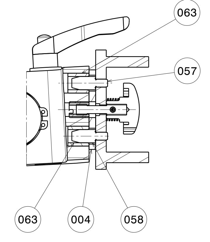
Coupe H-H Echelle : 3:5
