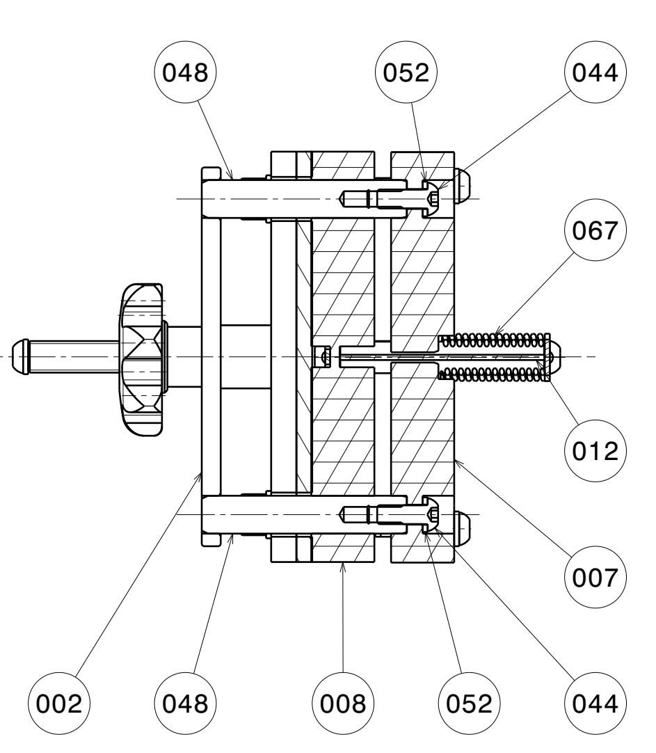
Coupe C-C Echelle : 3:5
