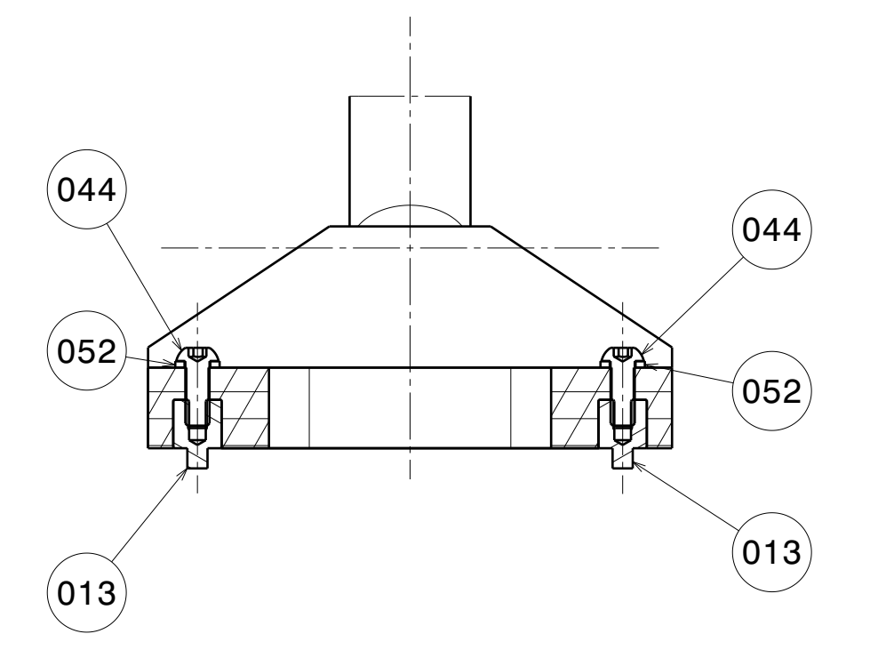
Coupe G-G Echelle : 3:5
