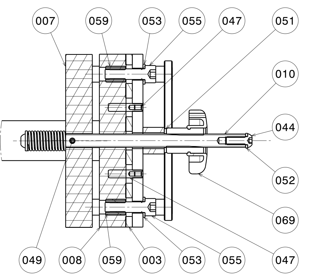
Coupe D-D Echelle : 3:5
