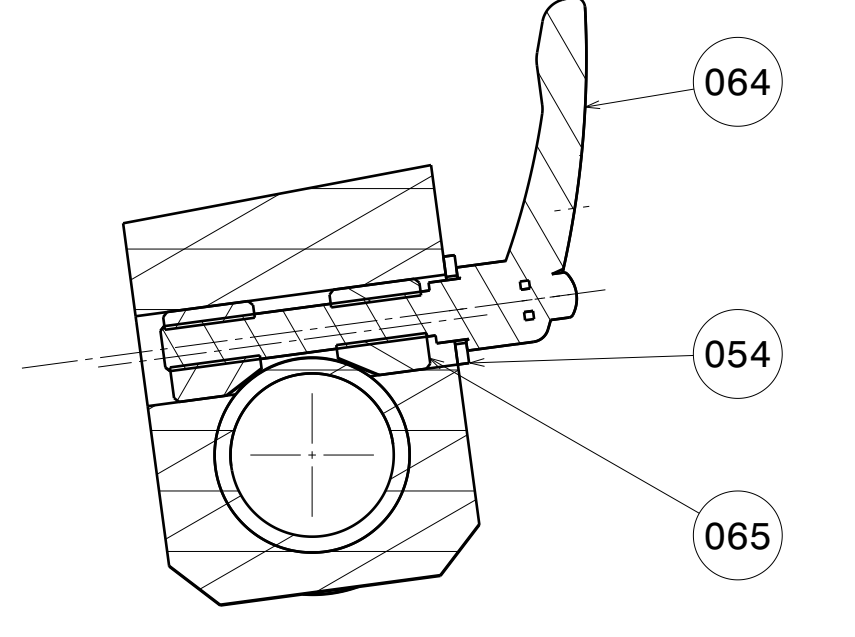
Coupe F-F Echelle : 3:5
