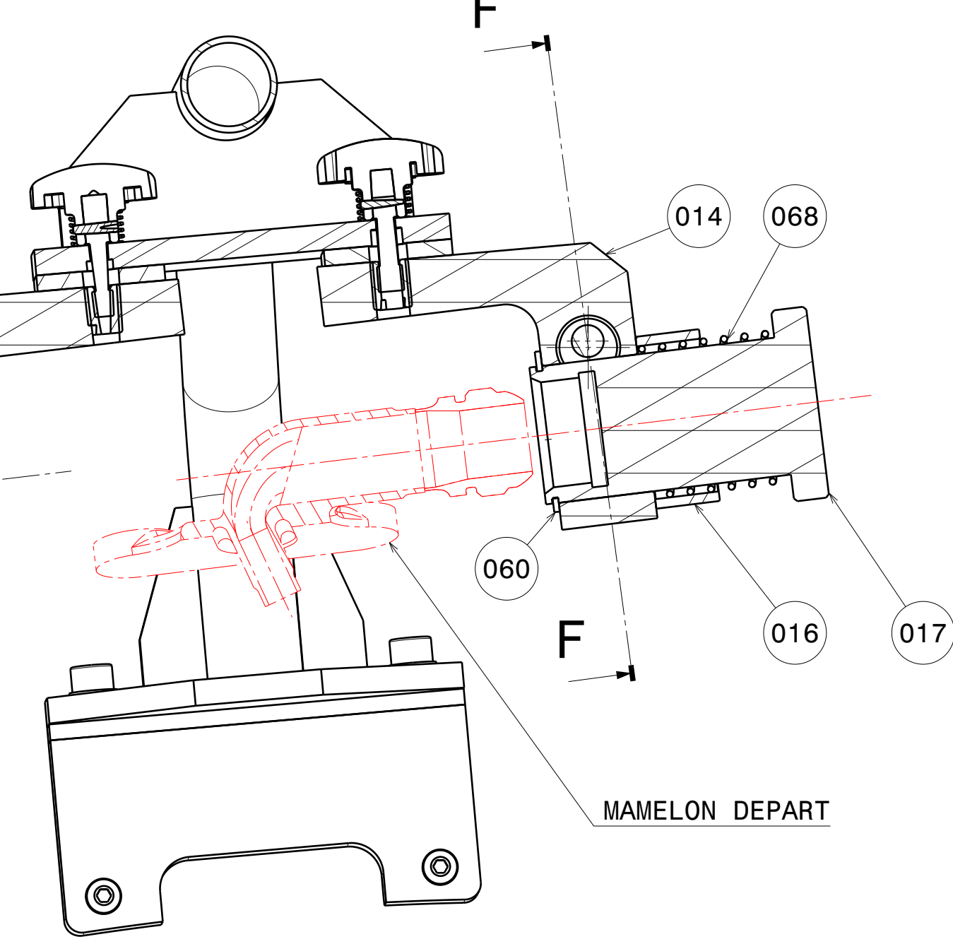
Coupe E-E Echelle : 3:5
