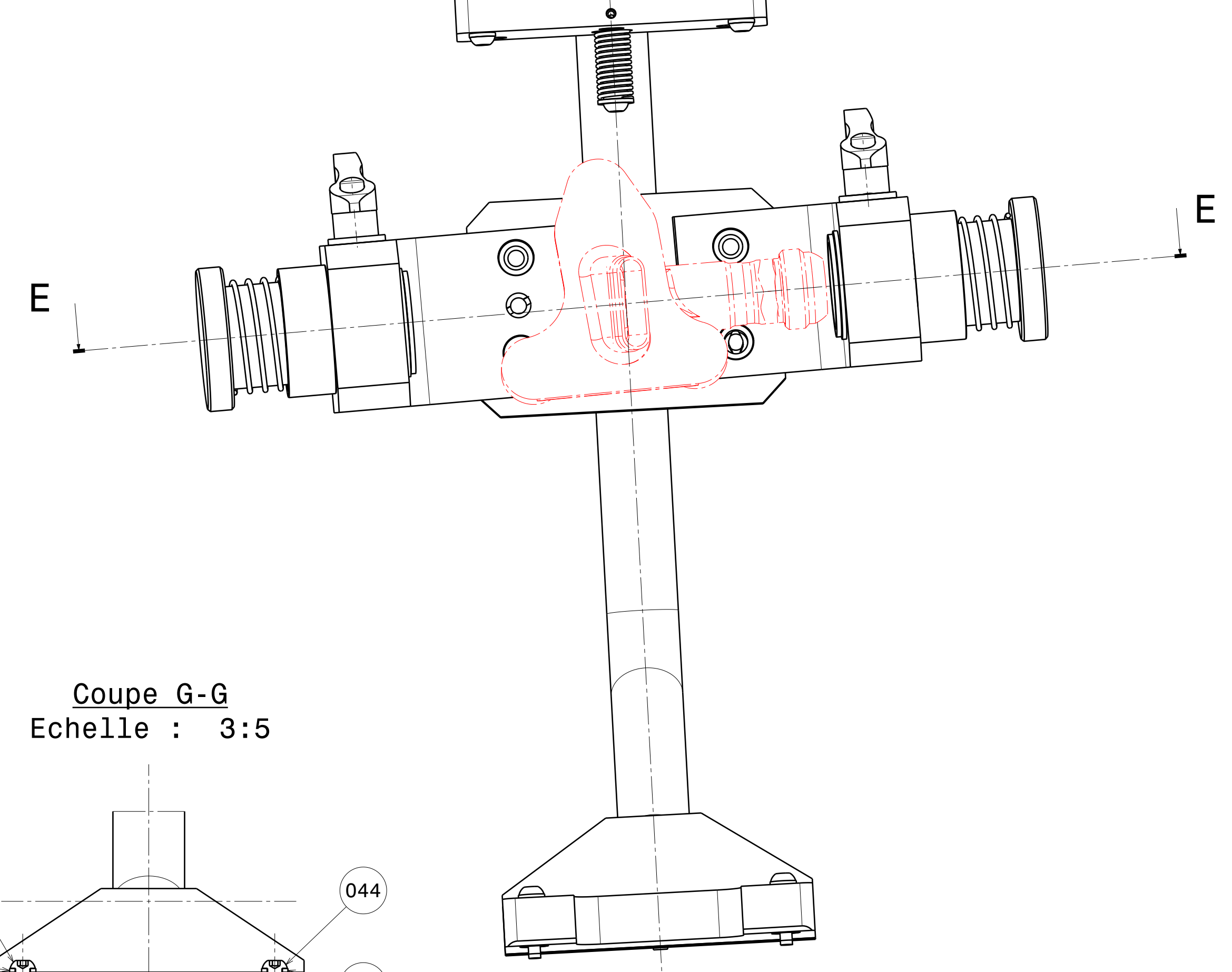
Vue auxiliaire J Echelle : 3:5
