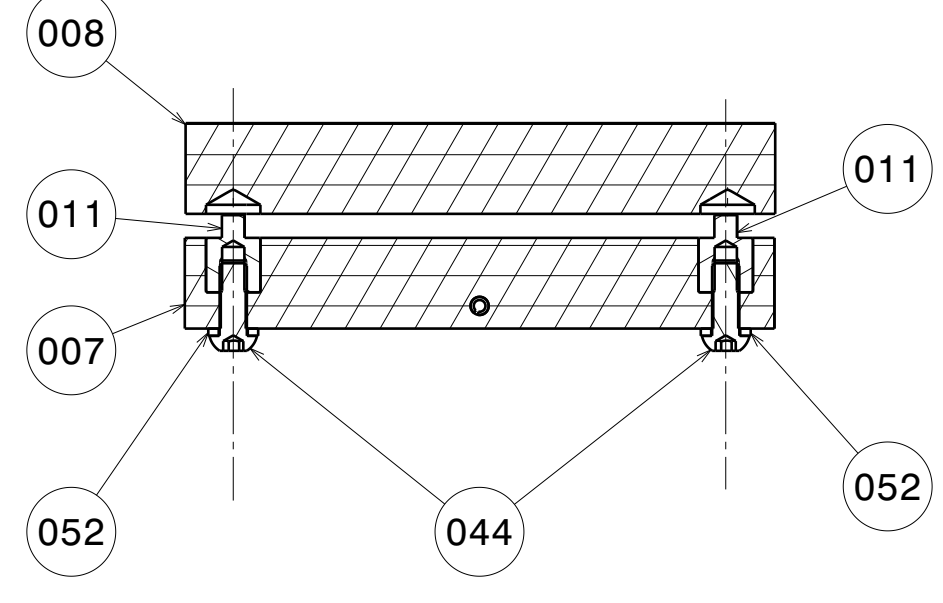
Coupe A-A Echelle : 3:5
