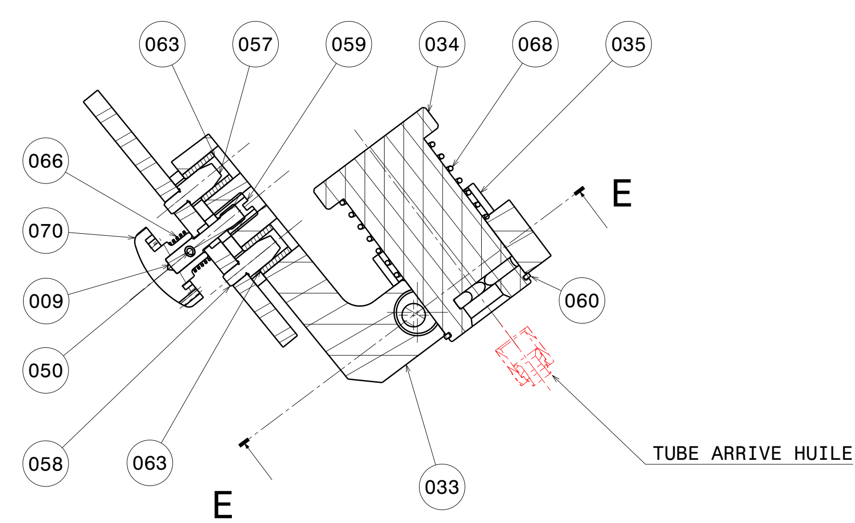
Coupe D-D Echelle : 3:5
