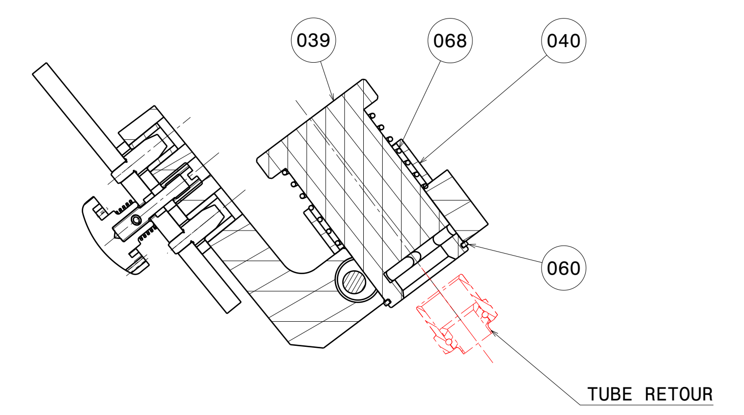
Coupe C-C Echelle : 3:5
