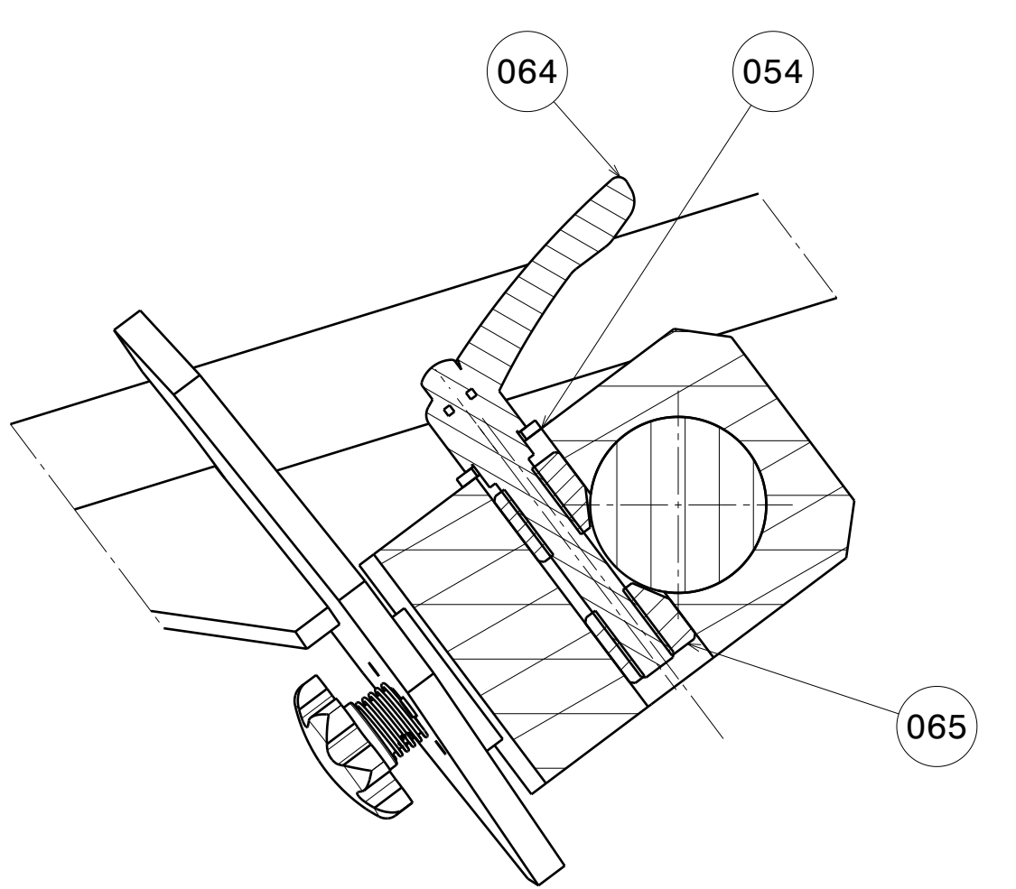
Coupe E-E Echelle : 3:5
