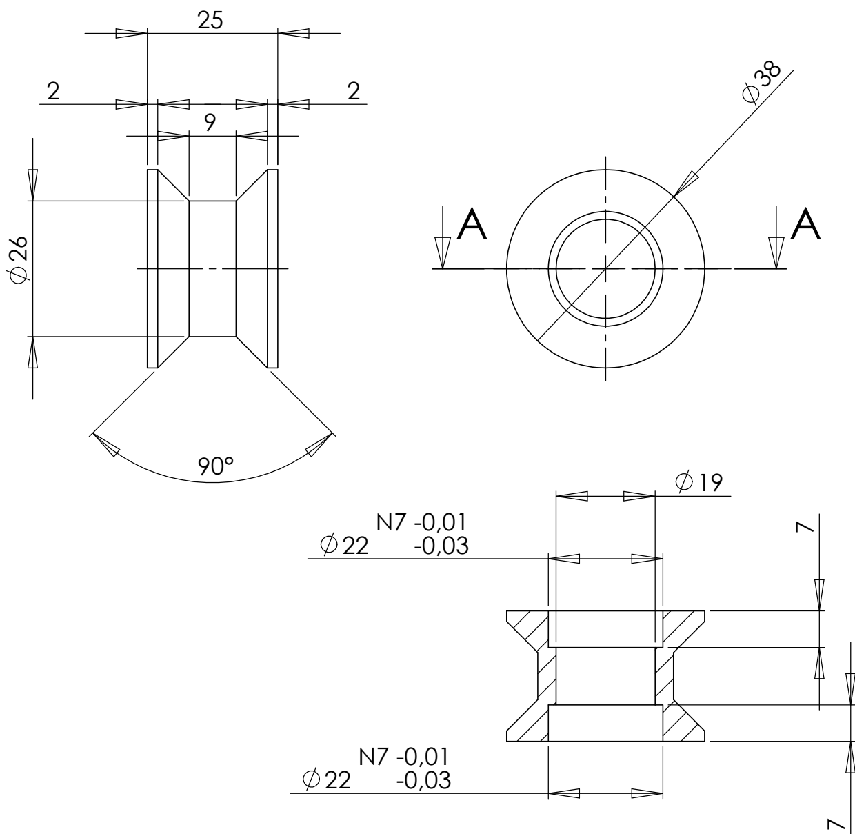
COUPE A-A
