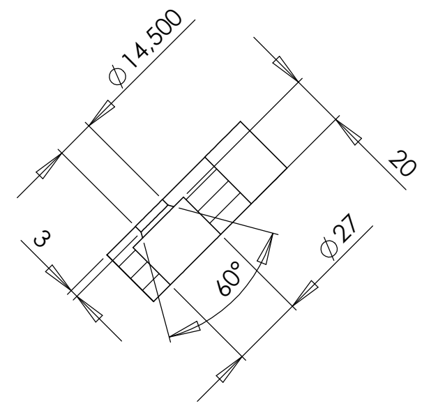
COUPE B-B
